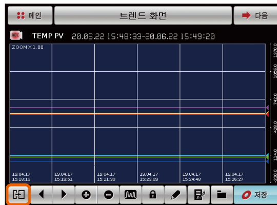
[그림 4-12] 전체 버튼 화면
