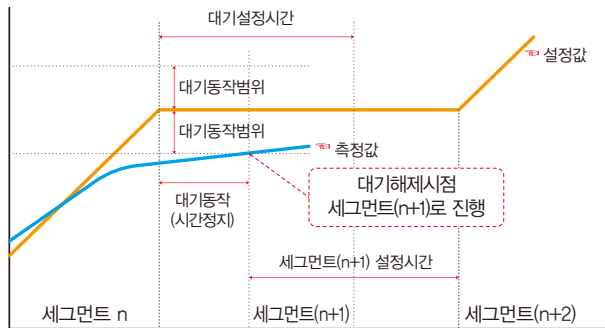
대기시간(WAIT TIME)이내에 대기동작 해제
