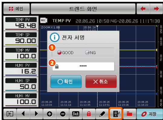
[그림 4-16] 전자 서명 버튼 화면
