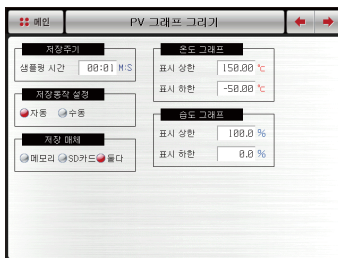
[그림 3-1] 그래프 & 저장 설정 제 1 화면
