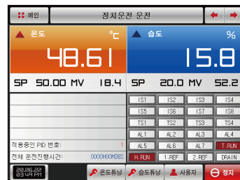
[그림 4-9] 정치운전 제 2 운전화면
