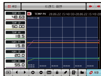
[그림 4-10] 정치운전 제 3 운전화면
