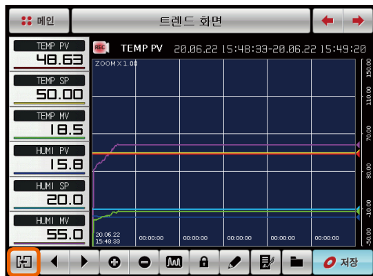
[그림 4-11] 부분 버튼 화면
