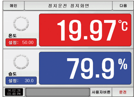
[그림 3-2] 정치운전 제 1 정치화면 (사용자 버튼)
