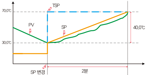
변화율(SLOPE) 동작
