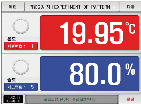
[그림 3-23] 프로그램운전 종료 화면
