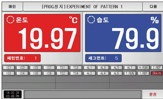
[그림 3-17] 프로그램운전 제 1 정지화면
