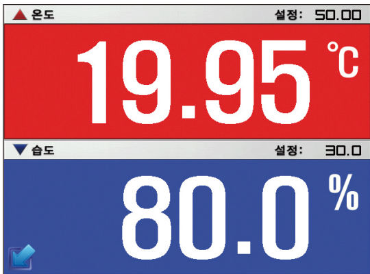
[그림 3-8] 정치운전 제 1 운전 확대 화면
